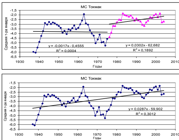
Рисунок 2 – Временной ход 11-летних январских температур для станции Токмак с графиками и уравнениями линейных трендов для периодов 1937–1975 и 1976–2004 гг. (верхний рисунок) и для всего периода в целом 1937–2004 гг. (нижний рисунок)
