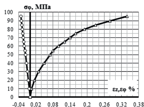
Рисунок 2 – Окружное растяжение (образец № 15)
