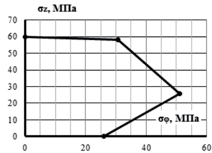
Рисунок 3 – Поверхность текучести
