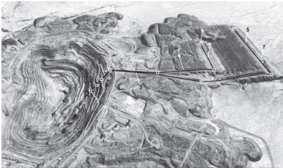
Рис. 1. Общий вид карьера «Мурунтау»: 1 – перегрузочные пункты; 2 – крутонаклонные конвейеры; 3 – конвейер КЛ-1; 4 – конвейер КЛ-2; 5 – отвальный конвейер породный; 6 – отвальный конвейер рудный; 7 – отвалообразователь породный ОШС-4000/125; 8 – отвалообразователь рудный ОШС-4000/125
