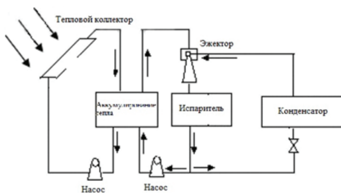
Рисунок 5 – Схема эжекторной системы
