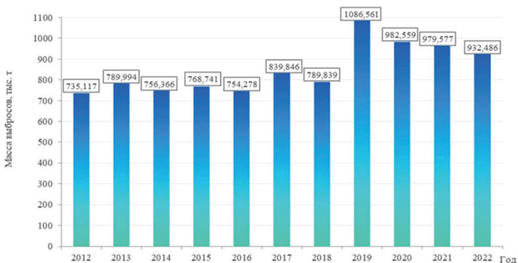
Рисунок 6 – Динамика выбросов метана от стационарных источников Кемеровской области – Кузбасса
