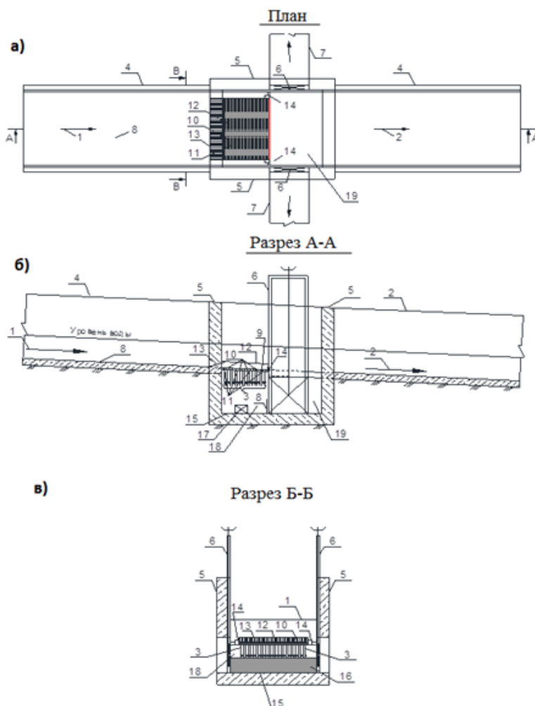
Рисунок 1 – Водовыпуск-стабилизатор расхода воды из каналов с бурным режимом течения: а – план водовыпуска из быстроточного канала; б – разрез А-А; в – разрез В-В. 1 – водный поток, 2 – транзитная часть, 3 – забираемая часть, 4 – канал, 5 – колодец, 6 – затворы водовыпуска, 7 – отводящие каналы, 8 – дно канала, 9 – решетка, 10 – пластины с наклонном обратно течению воды, 11 – щели, 12 – отсекатель воды, 13 – наклонная решетка, 14 – шарнир крепления, 15 – дно колодца, 16 – вертикальная стальная пластина для успокоения бурного режима воды, 17 – щиток для гидравлической очистки, 18 – отсек колодца, 19 – отсек для забора воды из колодца потребителям
