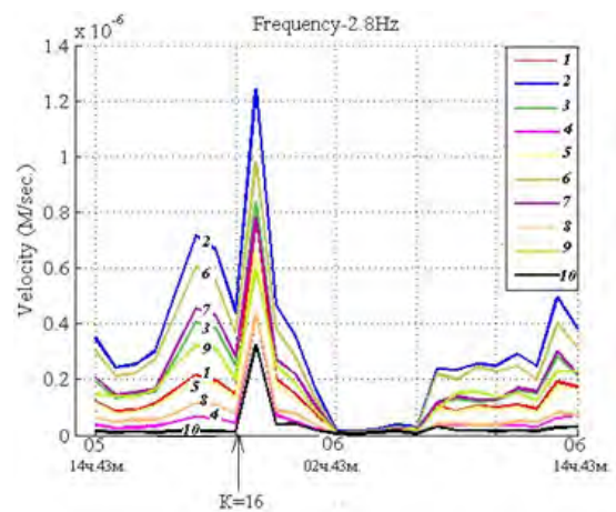
Рисунок 3 – Изменение во времени амплитуд колебаний шума на частоте 2,8 Гц с 14 ч 43 мин 5 октября по 14 ч 43 мин 6 октября. Стрелкой отмечен момент начала записи Нурина землетрясения на плотине
