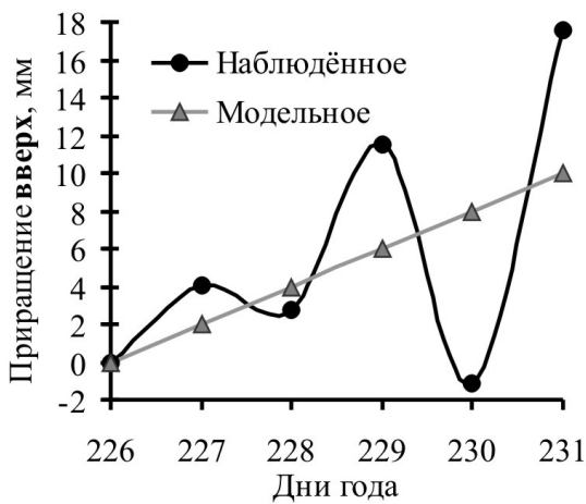
Рис. 5. Модельные и наблюдаемые графики посуточных приращений координат пункта IAT1 на юг, восток и вертикально вверх. Наблюдённые приращения компонент вычислены относительно статичного пространственного центра L и системы отсчета LNEH .
