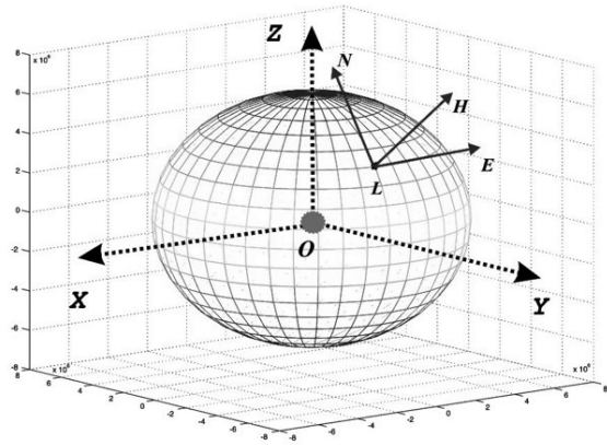
Рис. 4. Положение локальной системы координат ( LNEH ) относительно геоцентрической картезианской системы координат ( OXYZ ).
