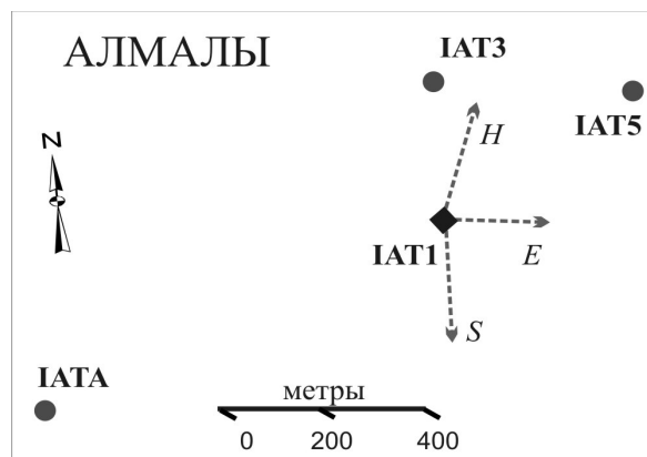
Рис. 2. Положение измеряемых реперов геодезической площадки Алмалы. На IAT1 установлена GPS антенна с 3D-корректором, на других тумбах антенны неподвижны.
