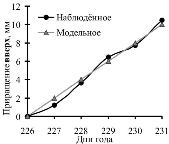
Рис. 7. Модельные и наблюдаемые графики посуточных приращений координат пункта IAT1 на юг, восток и вертикально вверх. Наблюдённые приращения компонент вычислены в стабилизированной системе отсчета LNEH' с динамично меняющимся пространственным центром L^{(i)} .
