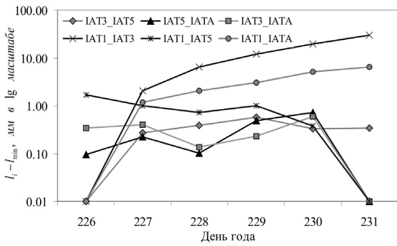
Рис. 3. Посуточные вариации длин шести базовых линий относительно минимальных значений ( \approx 0.01 ) в логарифмическом масштабе.
