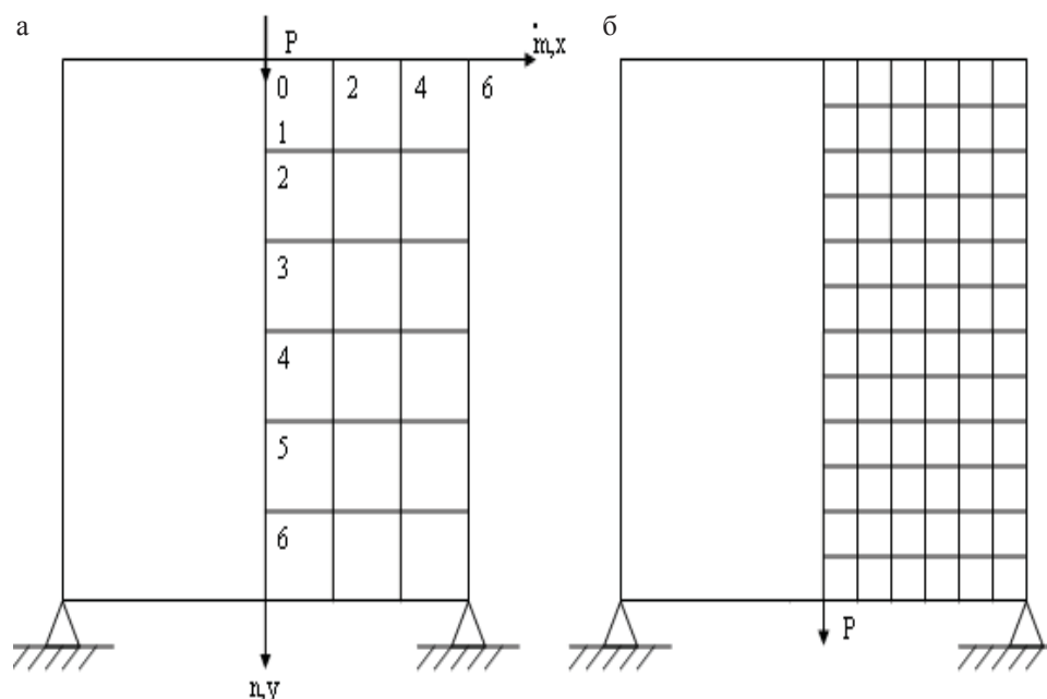
Рис. 5. Квадратная балка-стенка под действием сосредоточенной нагрузки, приложенной а – к верхней грани; б – к нижней грани.
